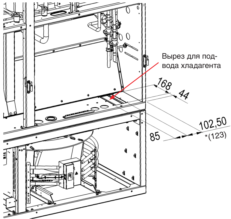
Типоразмеры 2 - 7
