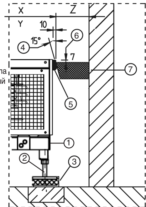
Детализация уплотнения при расстоянии Z \geq 100 мм
