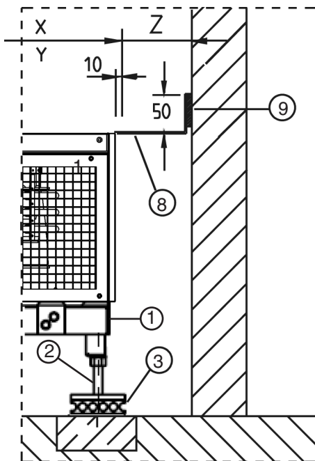
Детализация уплотнения при расстоянии Z < 100 мм
