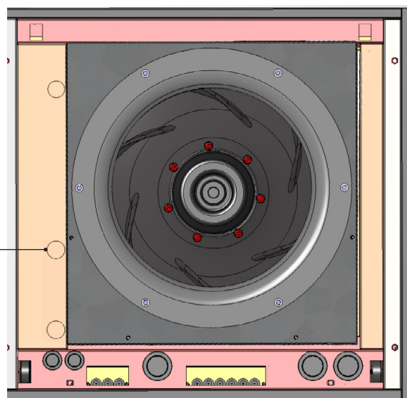
Вид блока вентиляторов сверху
