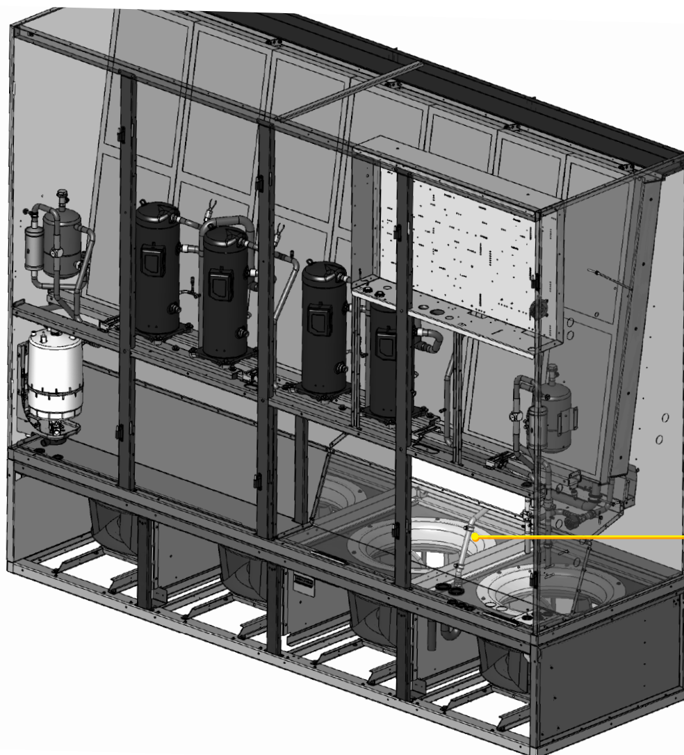
Патрубок для слива конденсата
