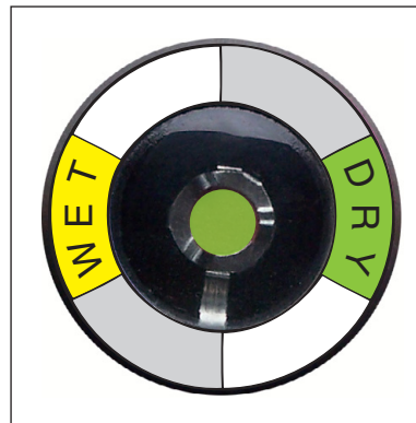
Смотровое стекло
