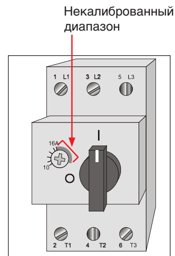
Включение выключателя питания
