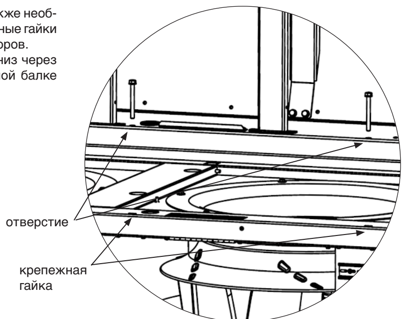
Подробный рисунок
