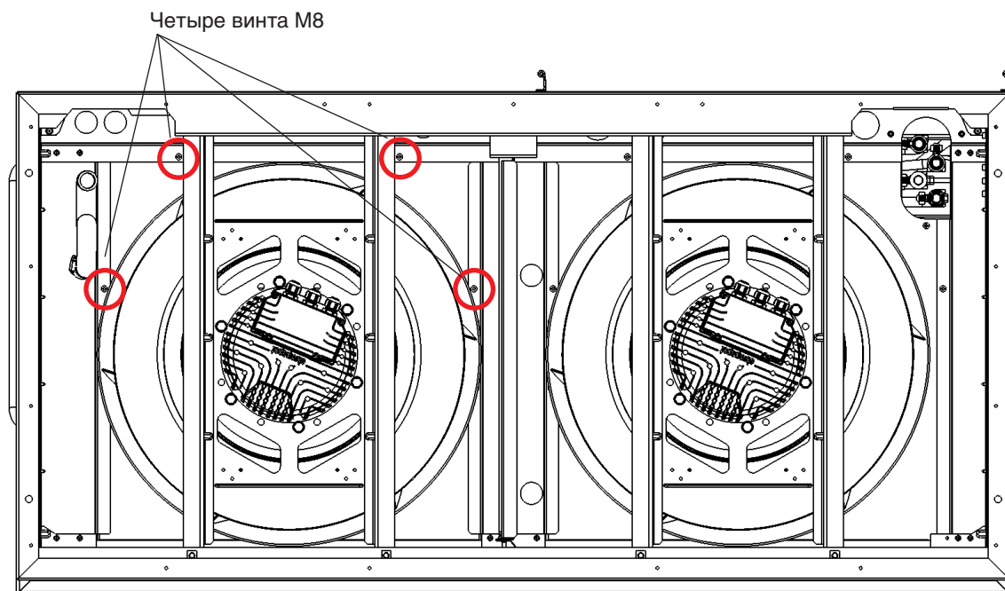
Вид блока вентиляторов снизу
