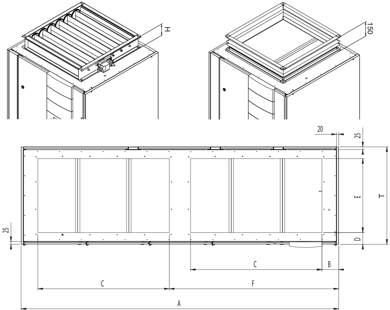
Переходная плита с воздушным клапаном
